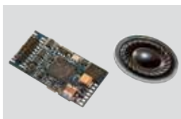
Decoder: 30 x 15,5 x 4,5 mm Lautsprecher: ø 23 mm
